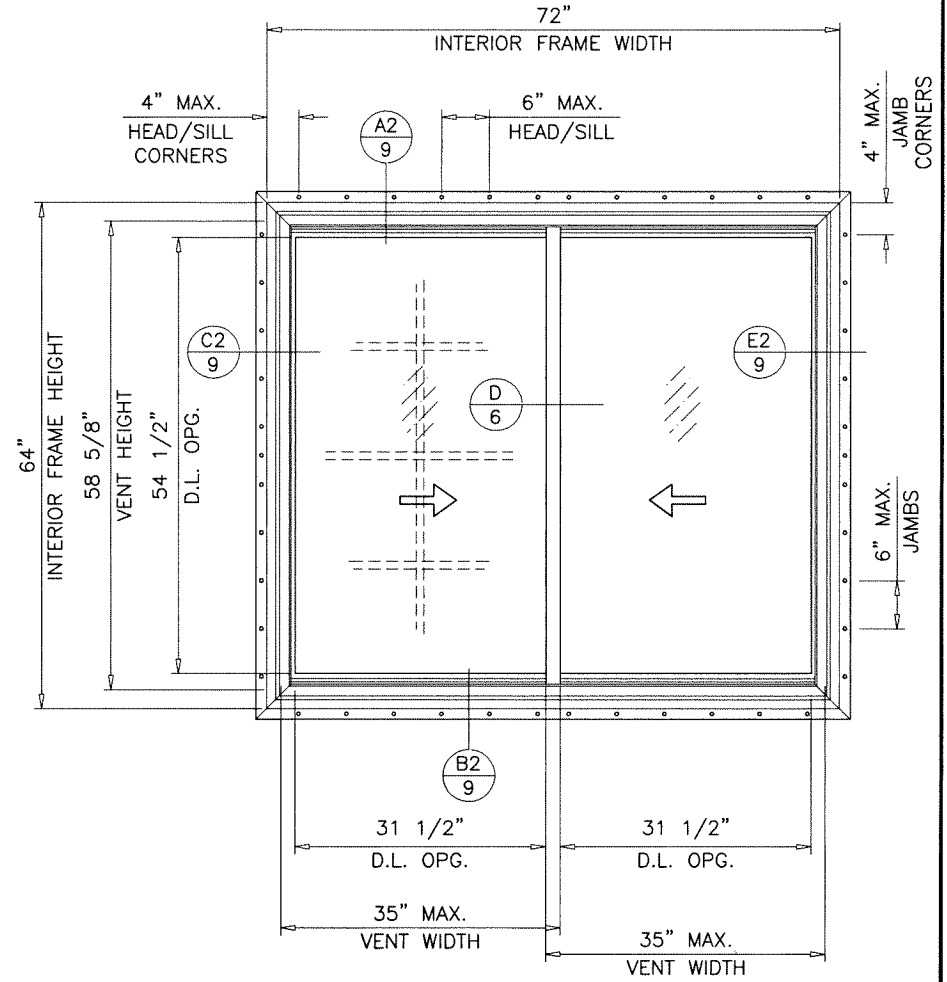
FIN FRAMES
