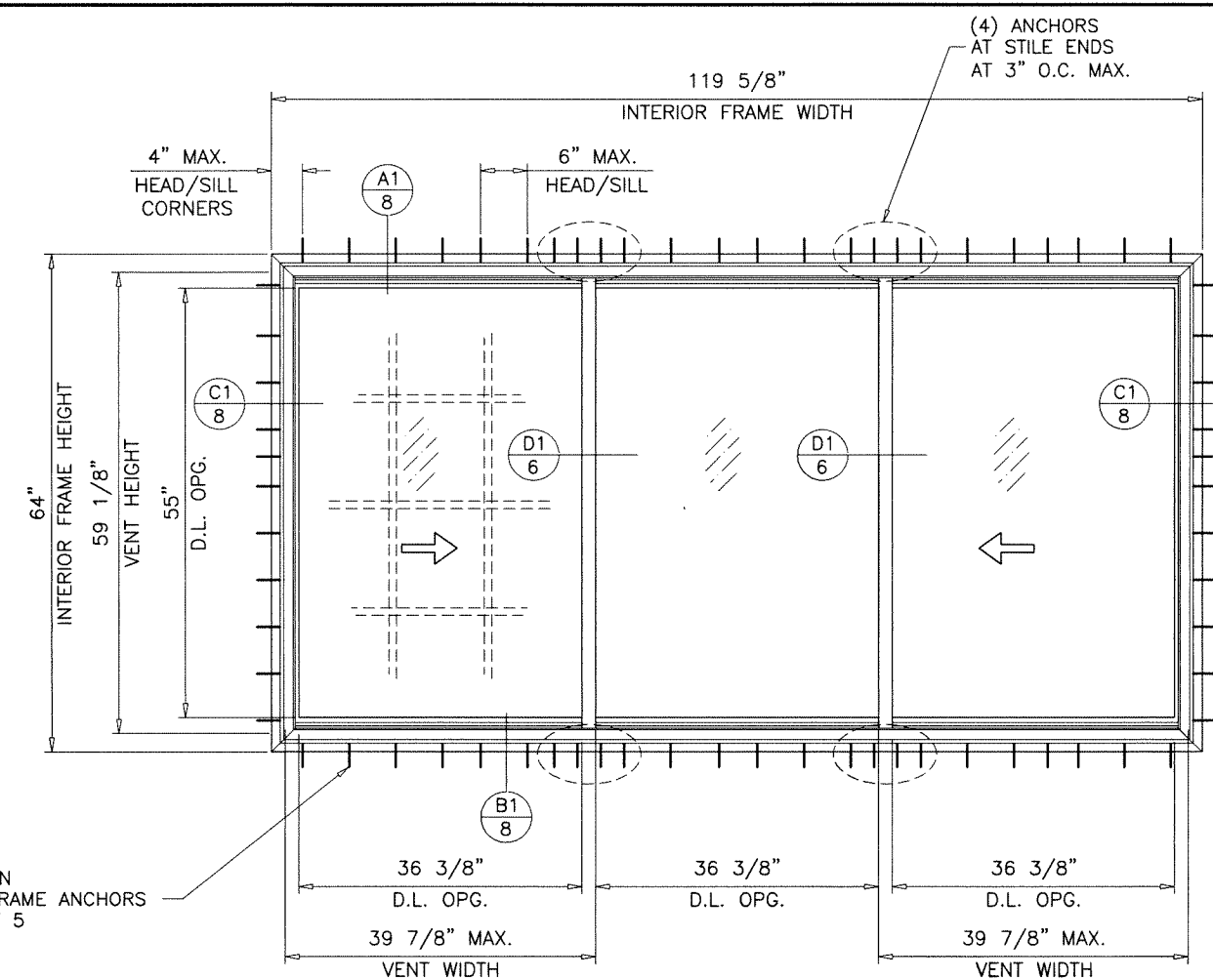
FLUSH FRAMES
