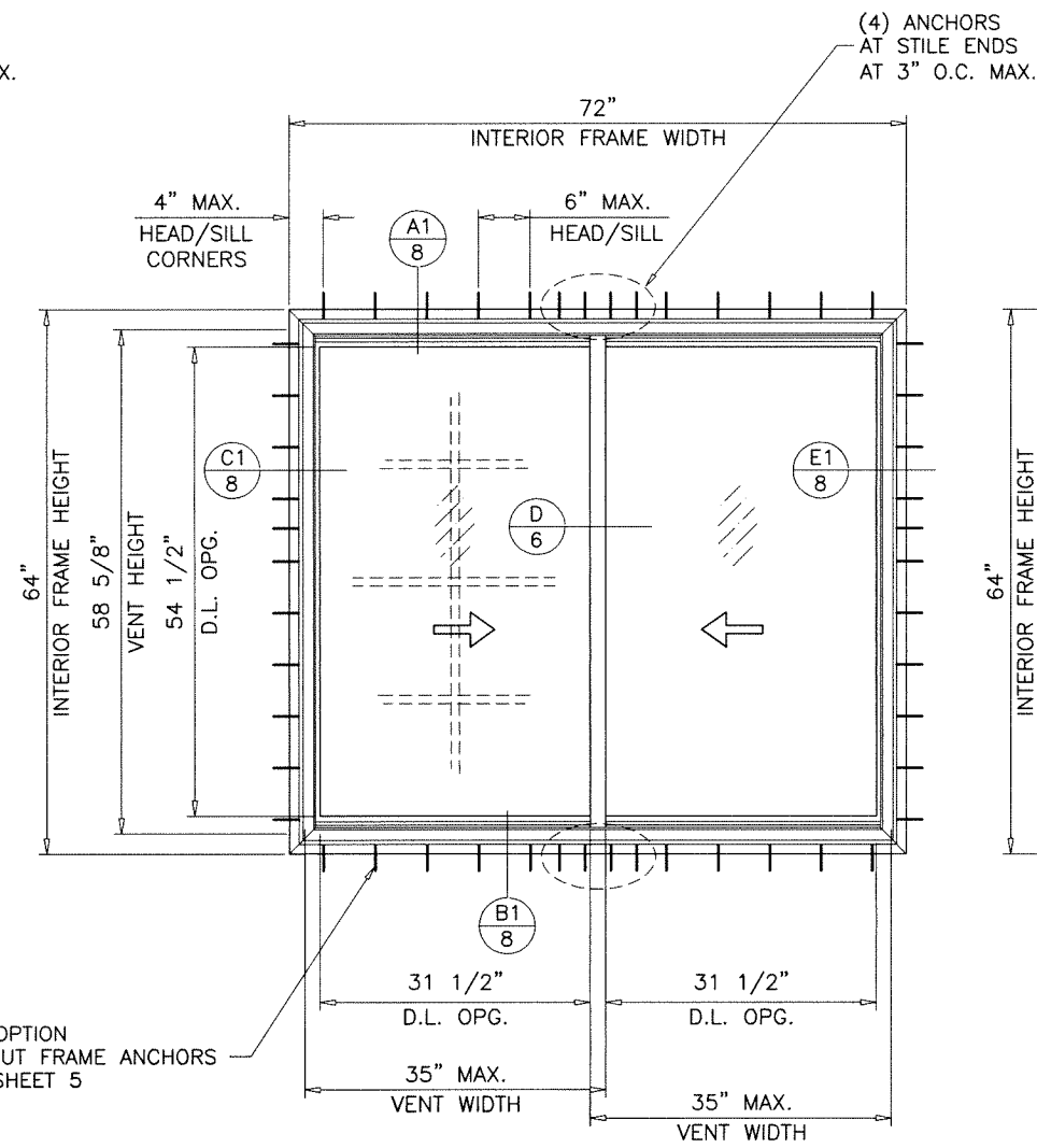
FLUSH FRAMES
