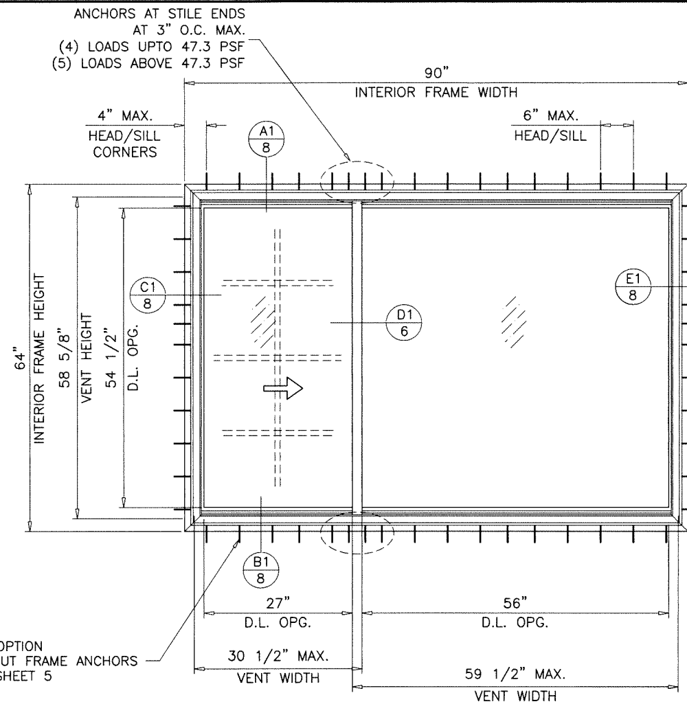
FLUSH FRAMES
