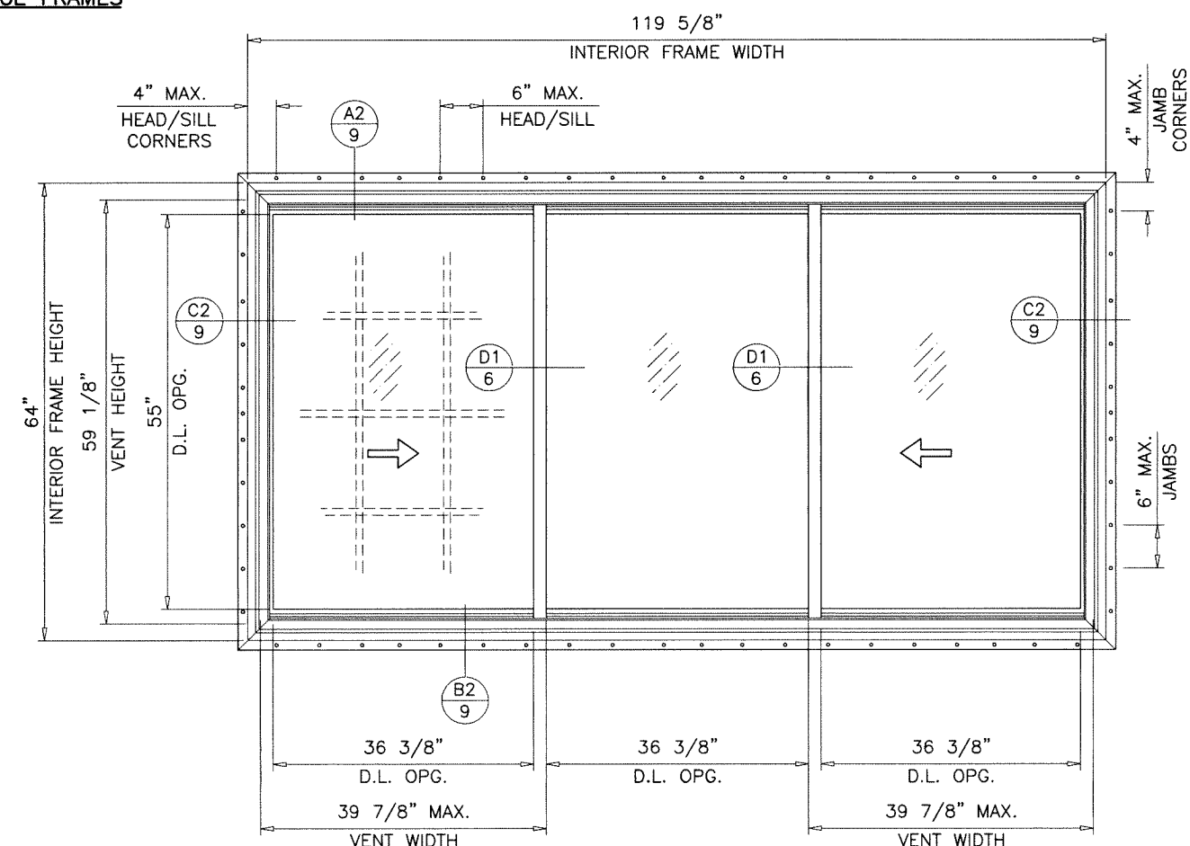
FIN FRAMES
